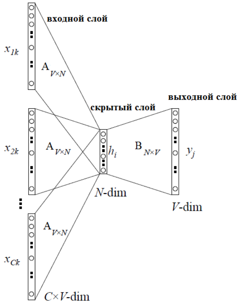
Рисунок 3. Архитектура метода SBOW для случая задания контекста с помощью нескольких слов.
