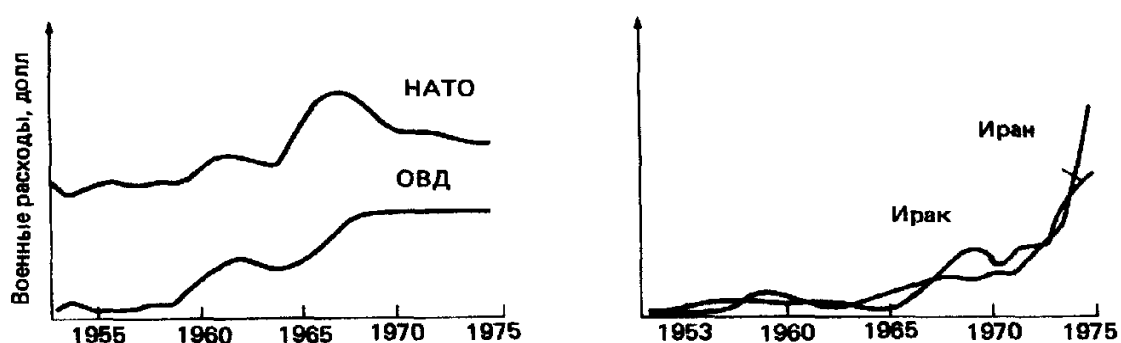
Рис. 1. Графическая интерпретация модели.
