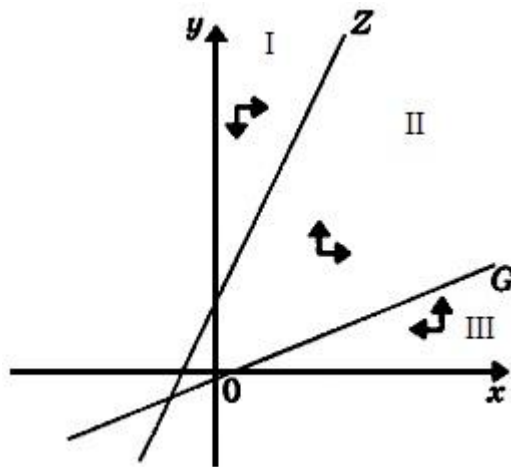
Рис.4. Точка равновесия в третьем квадранте .
