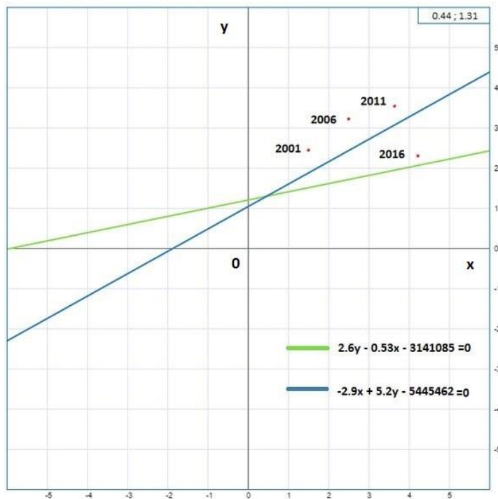
Рисунок 6. График уравнений системы.
