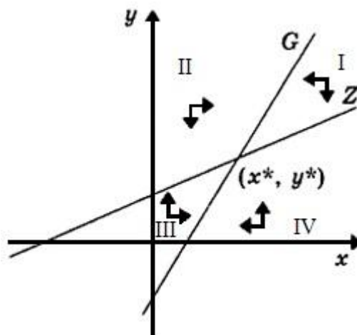
Рис.3. Точка равновесия в первом квадранте
