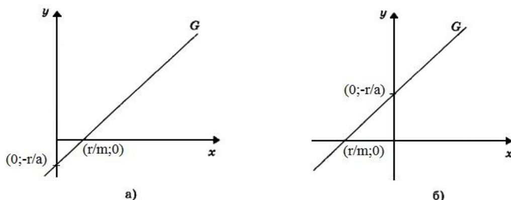
Рис.2. Геометрическая интерпретация уравнения (5): а) r > 0 ; б) r < 0 .
