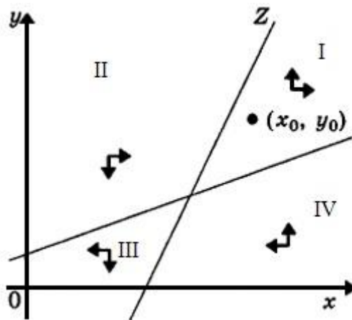
Рис.5. Поведение системы при r < 0 или (и) s < 0 .
