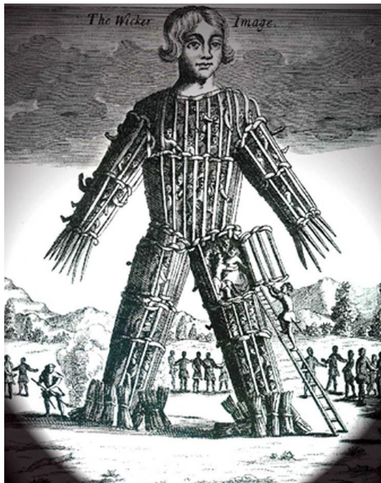
Рис. 1. Человеческие жертвоприношения
