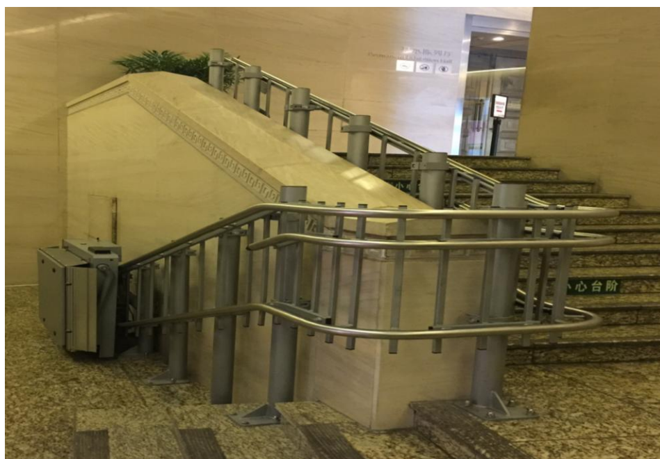
Фото 11. Механизм для перемещения колясок, установленный на внутренней лестнице международного аэропорта Пекина
