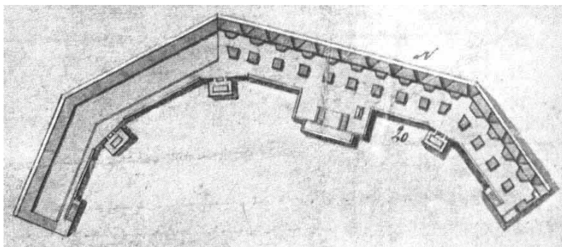
Рис. 1. План Двойной Южной батареи
