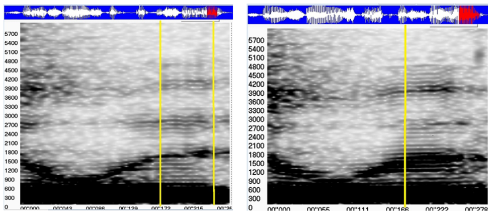
Рис. 3.3.1. Спектральное отображение сочетаний [o:ðə] и [o:ð]. (Диктор 2).
