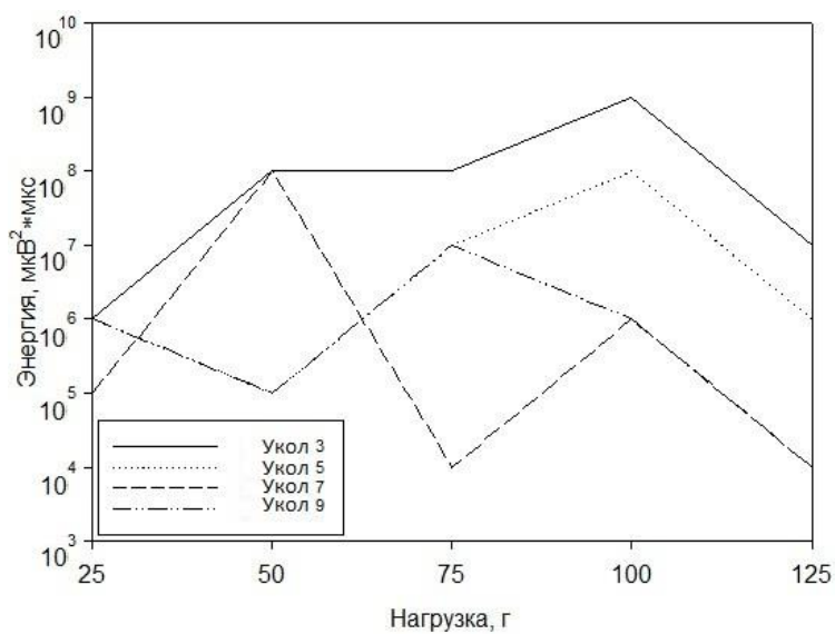
Рис. 3.3 Акустическая эмиссия.
