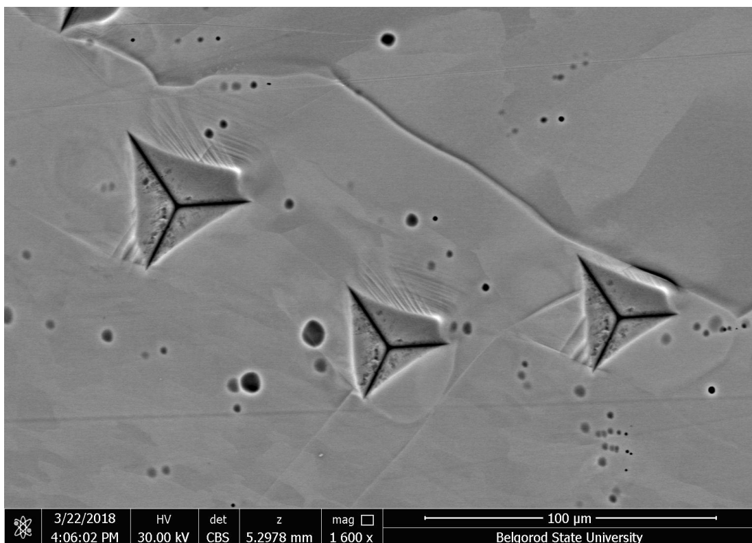
Рис. 3.6 Остаточные двойники в \alpha -титане при индентировании
