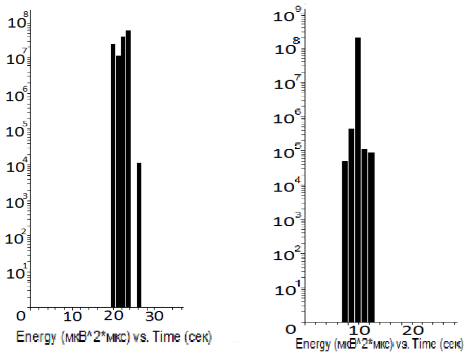
Рис. 3.2 Акустическая эмиссия в \alpha -титане при индентировании с нагрузкой а) 50 грамм; б) 75 грамм.
