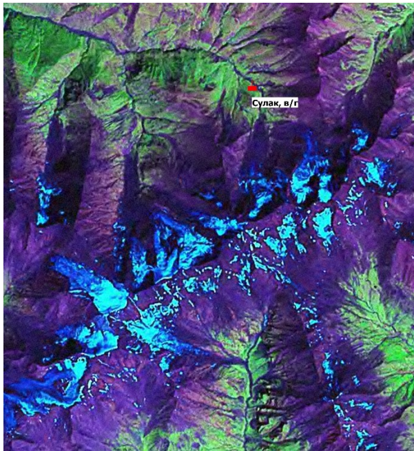
Рис. 4. Основные ледники Богосского хребта: а) на космоснимке; б) картосхеме [11]
