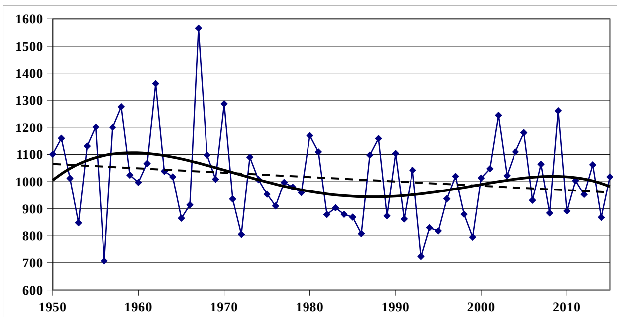
Рис. 3. Изменение величины годовых осадков за 1950-2015 гг. (м/с «Сулак, высокогорная»)
