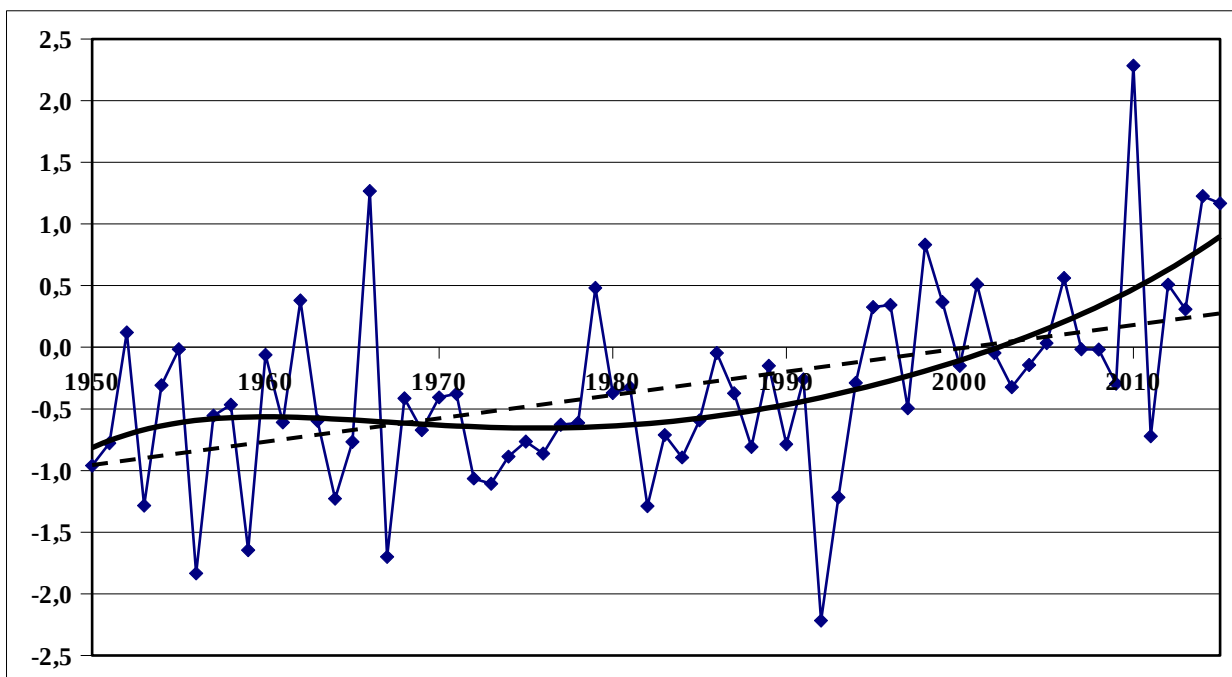
Рис. 2. Изменение средней годовой температуры воздуха за 1950-2015 гг. (м/с «Сулак, высокогорная»)
