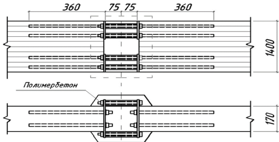
Рисунок 1.10 – Изгибаемый стык типа ПИ-1
