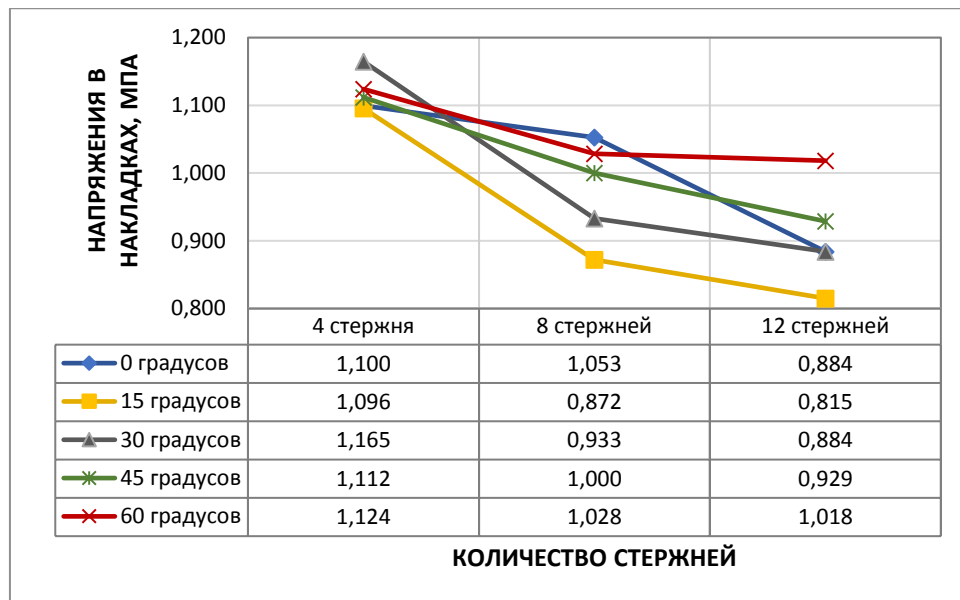
Рисунок 4.7 – График зависимости максимальных напряжений в накладках от угла вклейки и количества нагелей
