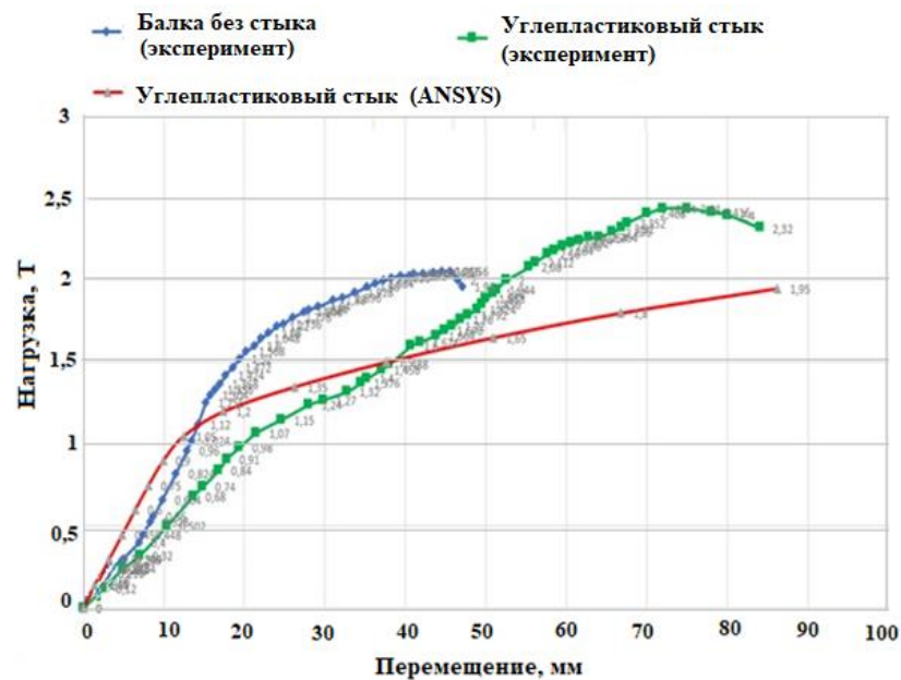
Рисунок 4.29 – Графики зависимости перемещений свободного конца балки от нагрузки в вычислительных и натуральных экспериментах
