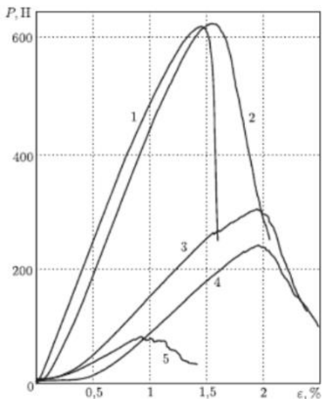
Рисунок 2.16 – Диаграмма растяжения для образцов из базальта
