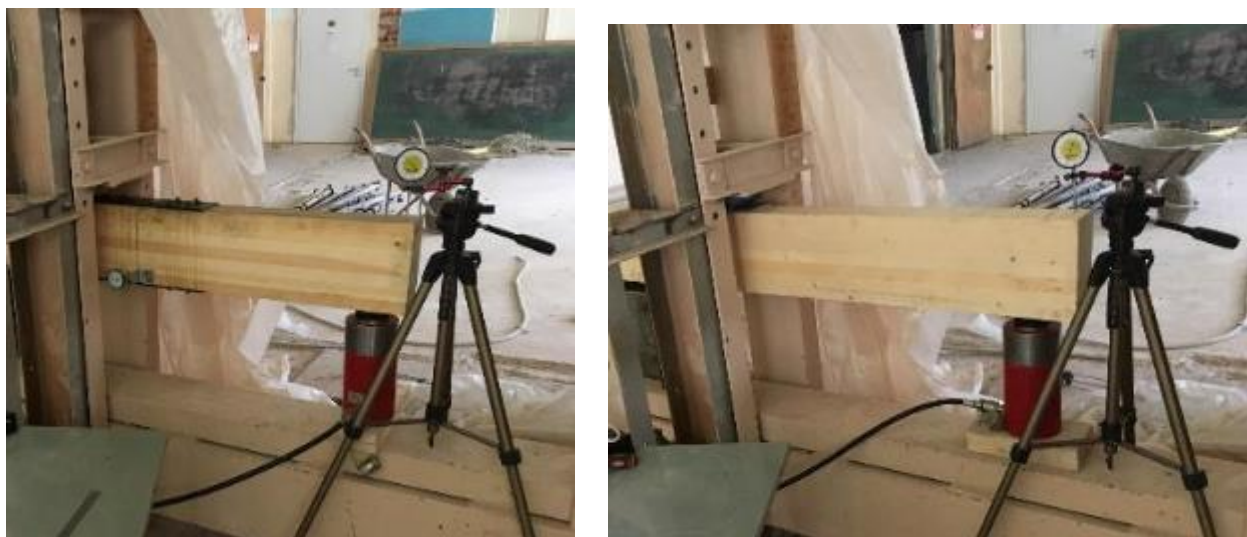
Рисунок 4.26 – Балки со стыком и без стыка на испытательном стенде
