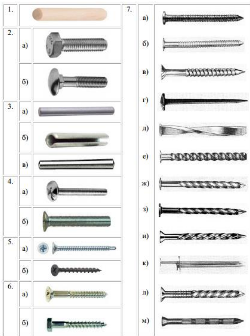
Рисунок 1.1 – Основные виды нагелей, используемые в соединениях конструкций из древесины (1 – дубовый нагель, 2 – болты, 3 – штифты, 4 – винты, 5 – самонарезающие шурупы, 6 – обыкновенные шурупы, 7 – гвозди)
