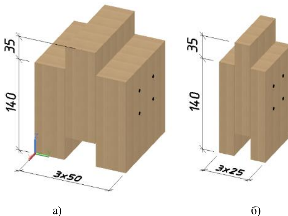
Рисунок 3.4 – Схема образцов: а) с толщиной доски 50 мм; б) с толщиной доски 25 мм
