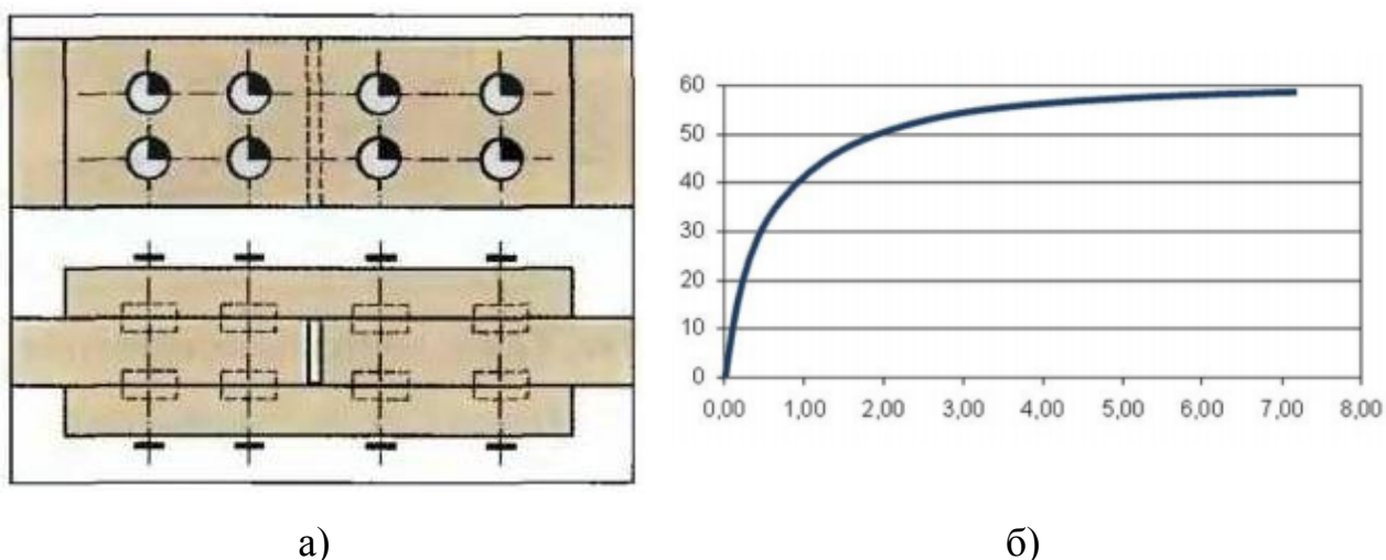
Рисунок 1.2 – Нагельное соединение
