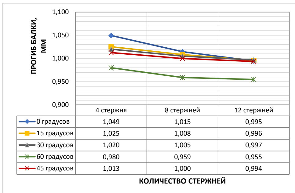
Рисунок 4.8 – Предельные вертикальные перемещения (прогибы)
