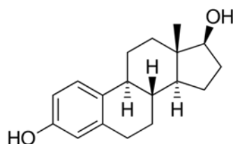
Рисунок 4 – Структурная формула эстрадиола
