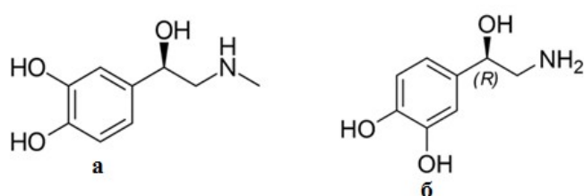
Рисунок 11 – Структура молекул адреналина (а) и норадреналина (б)
