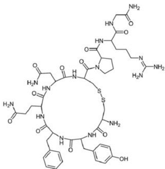
Рисунок 16 – Структурная формула вазопрессина
