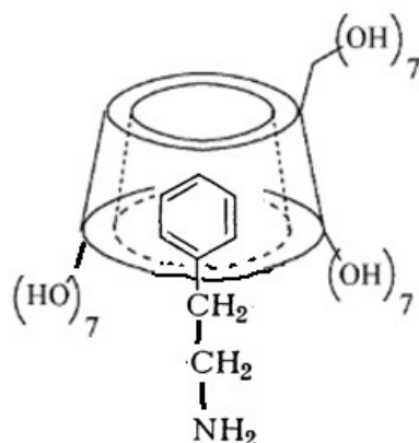
Рисунок 27 - Вариант комплекса \beta -циклодекстрин : 2-фенилэтиламин
